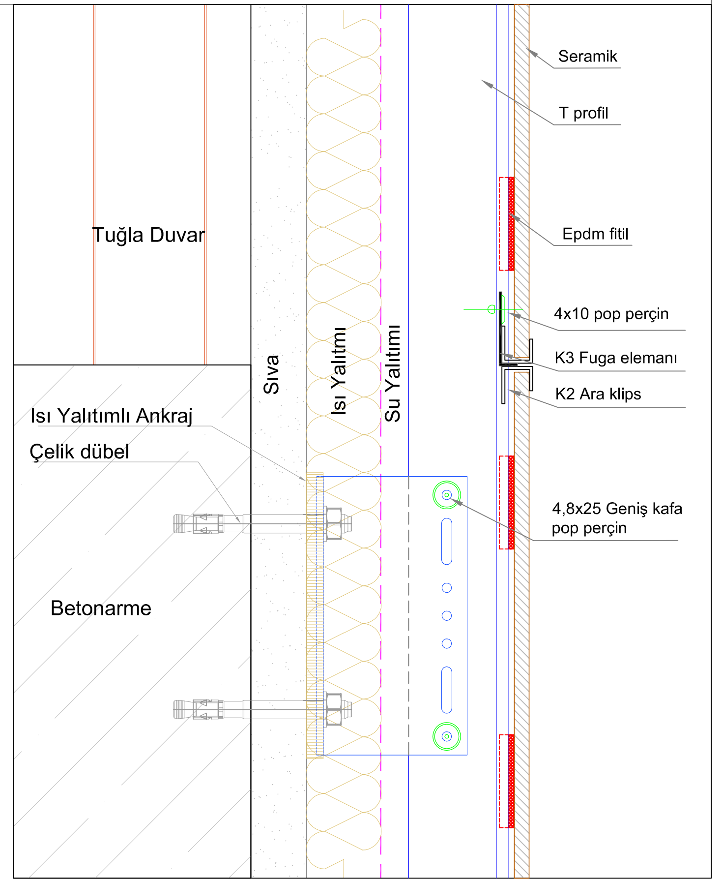
DETAY 4B
