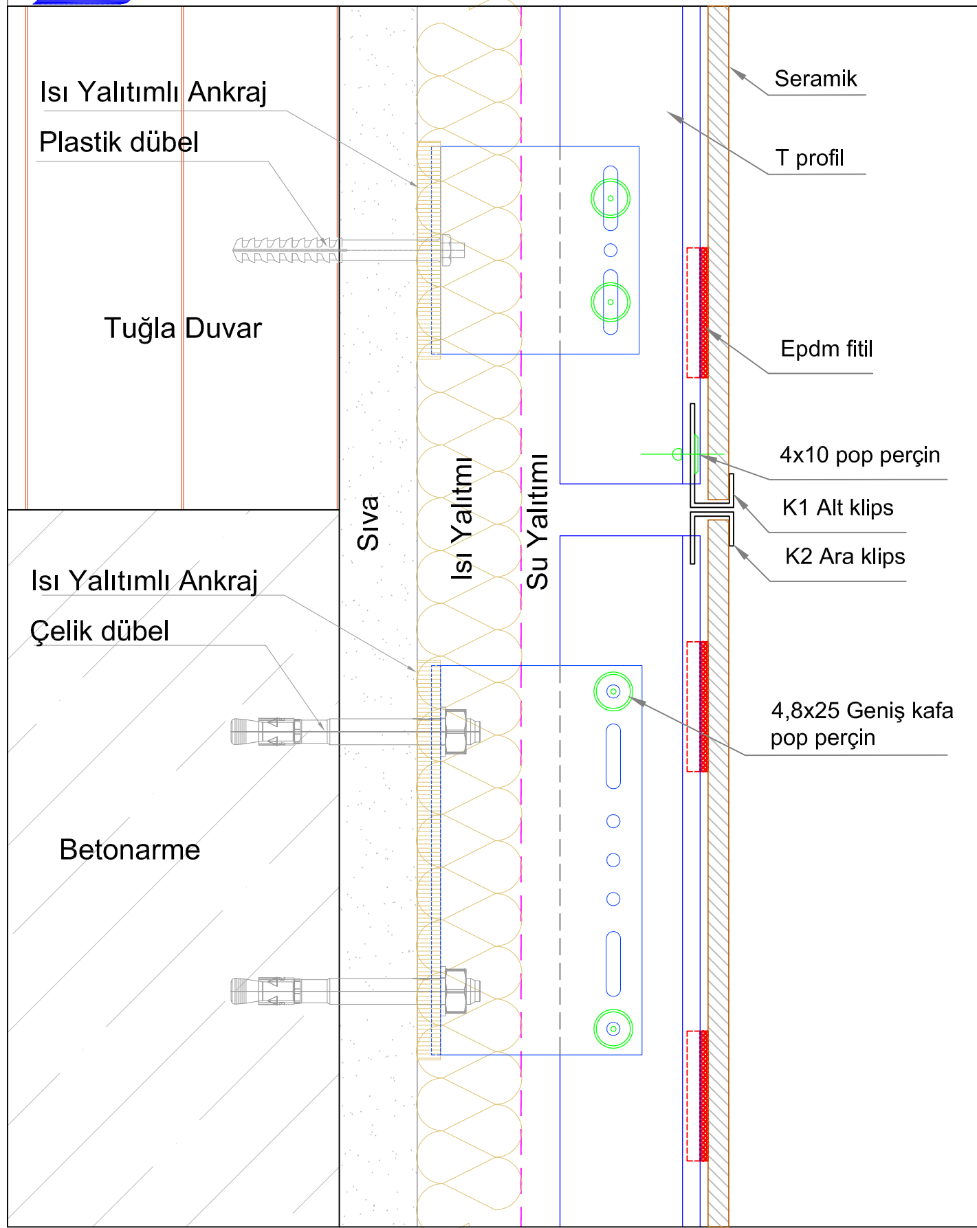
DETAY 4A
