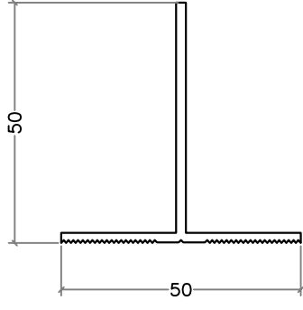
T Profil (50x50)
