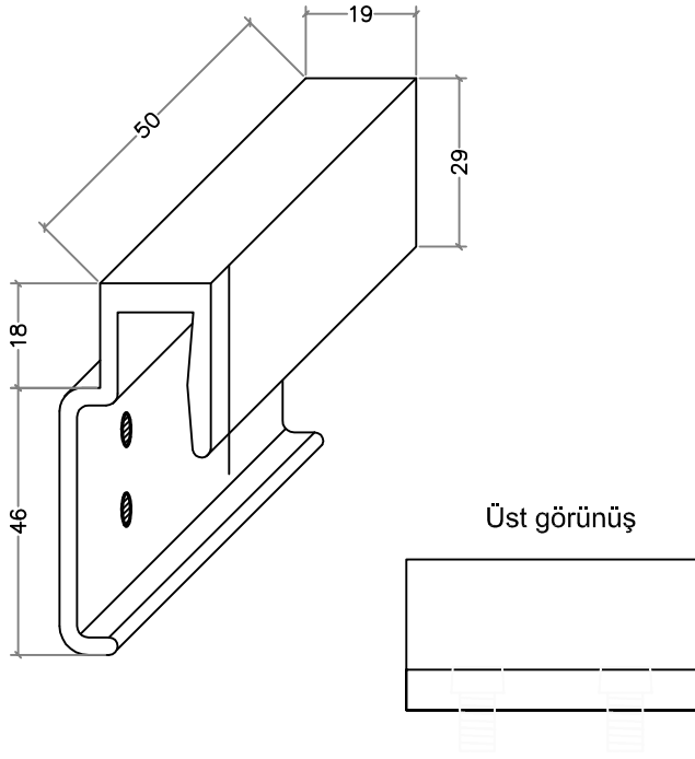
Alt Klips (Adet olarak temin edilir.)
