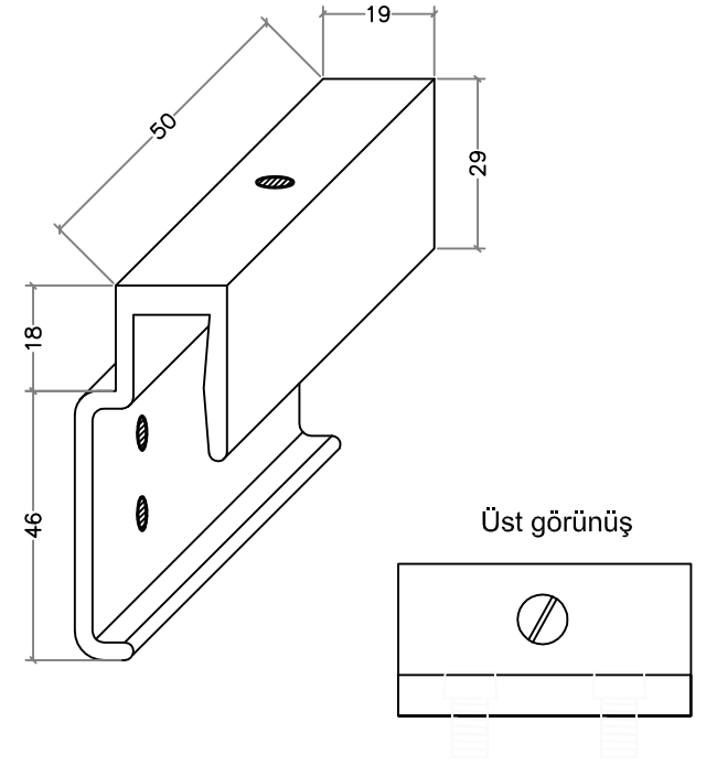
Üst Klips (Adet olarak temin edilir.)
