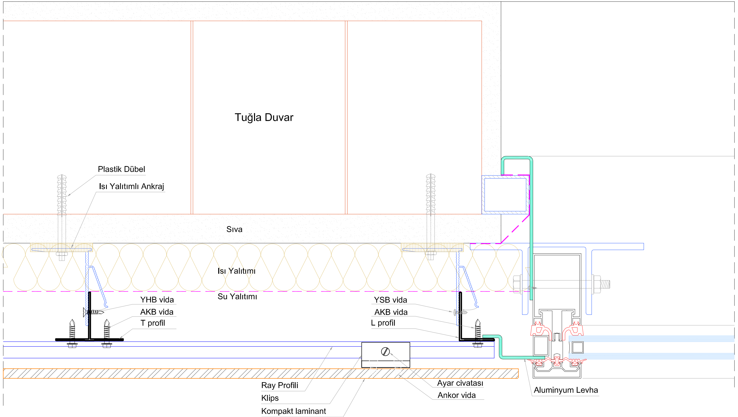
DETAY A
