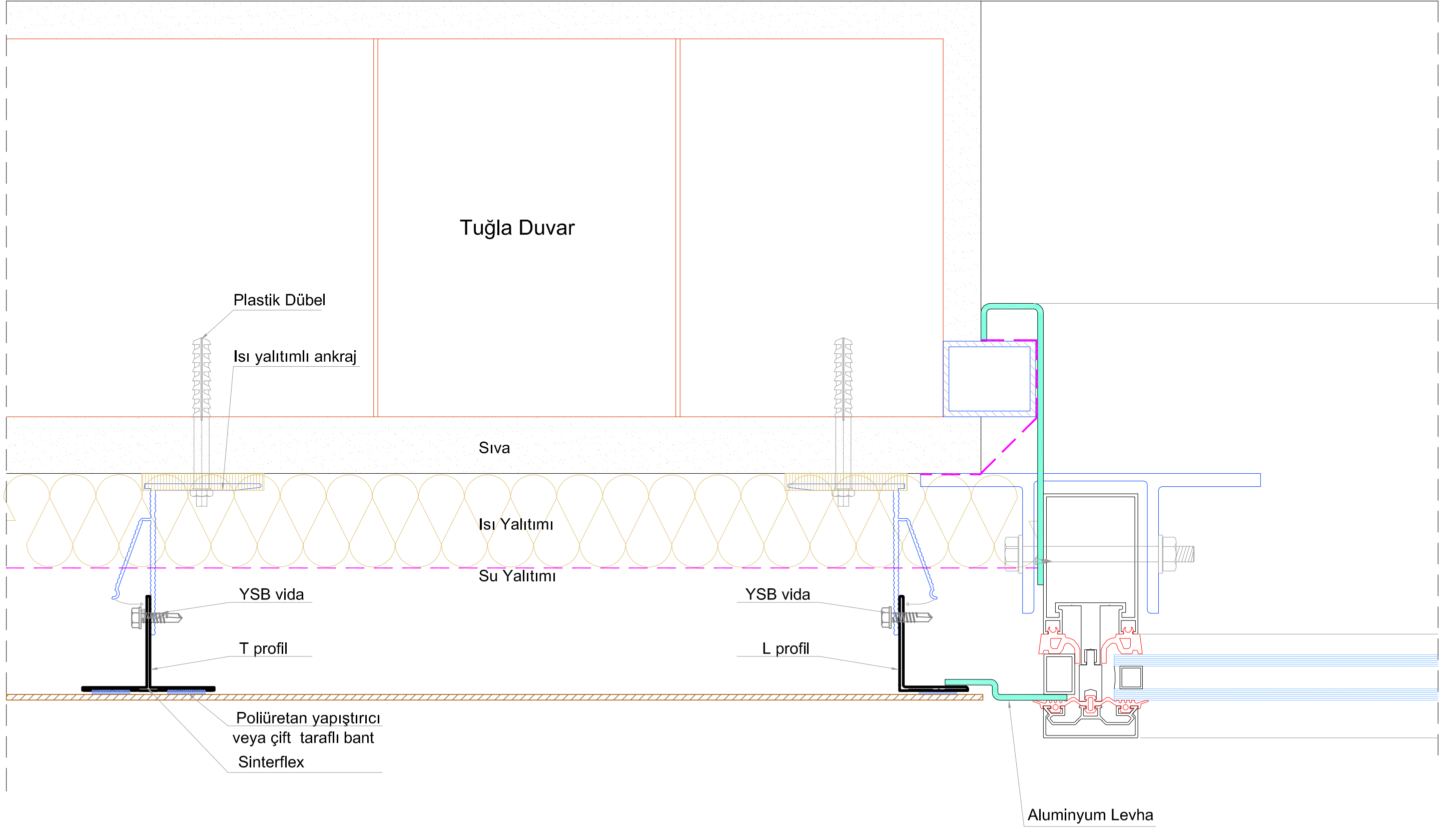
DETAY A
